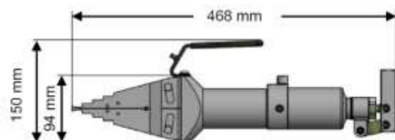
WYMIARY NARZĘDZIA: CAŁKOWICIE ZAMKNIĘTY
